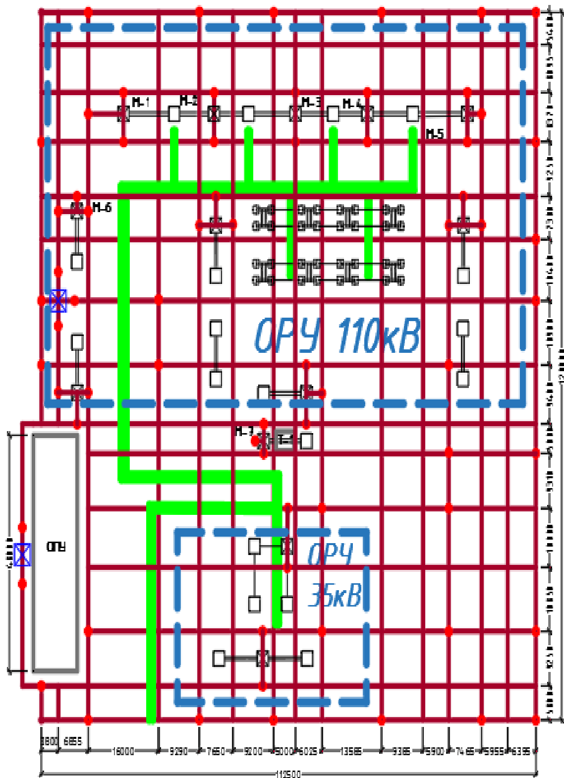
Рис. 2. Модель ЗУ ПС 110 кВ «Раззакова»
